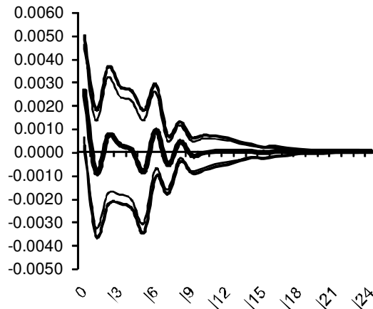
Respuesta ? PIB a ? GIGNC
