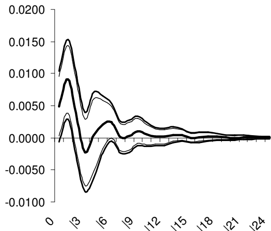
Respuesta \Delta P_{\text{Gasolina}} a \Delta \text{Vol}
