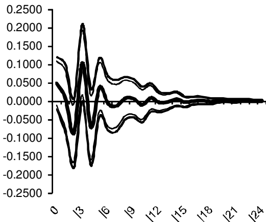
Respuesta ? GIGNC a ? ppos
