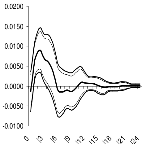
Respuesta \Delta P_{\text{Gasolina}} a \Delta p
