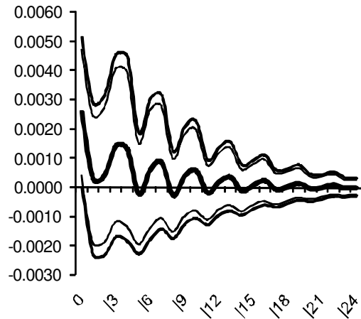
Respuesta ? PIB a ? ti_ind
